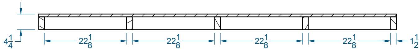
SECTION A-A
